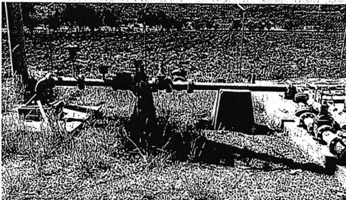
Tren de descarga en 4" pozo Joaquín Amaro.
