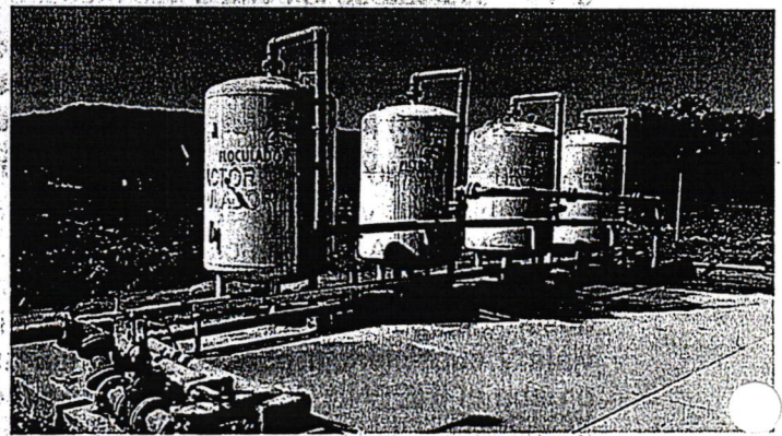
Planta Potabilizadora
